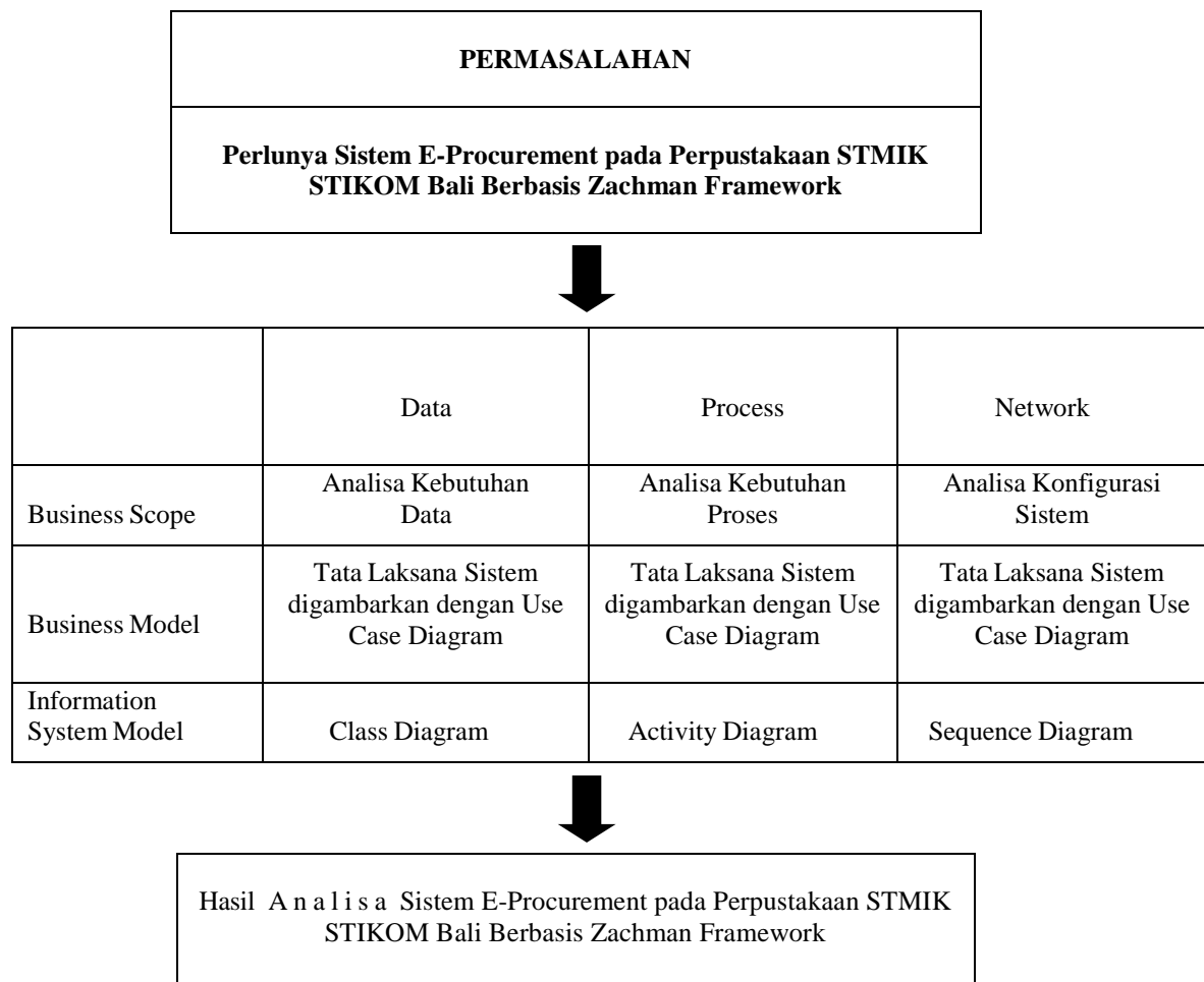
Gambar 2. Kerangka Arsitektur dengan Zachman Framework
