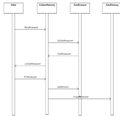
Sequence Diagram Penentuan Pemenang
